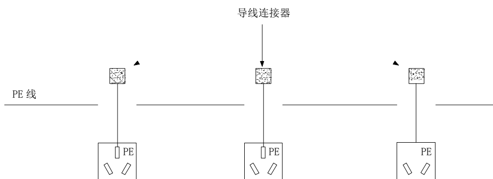
图 20.1.3b PE 线不串联连接的做法
